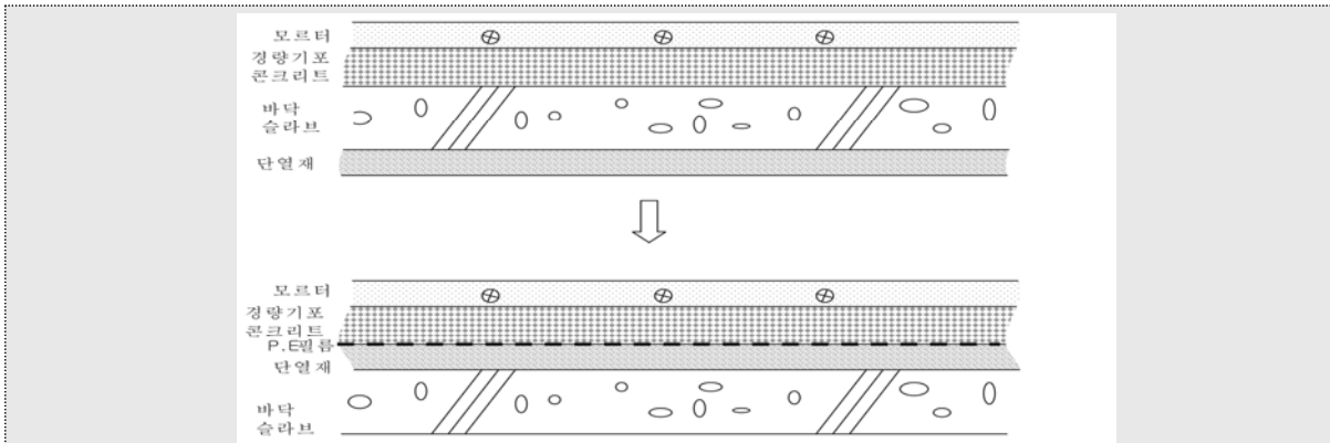
<최하층 온돌의 단열재 설치 위치 예시도>
