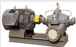
양쪽 흡입 벌루트 펌프
