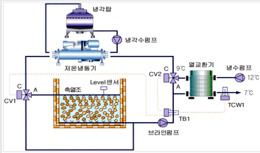
[빙축열 시스템]
