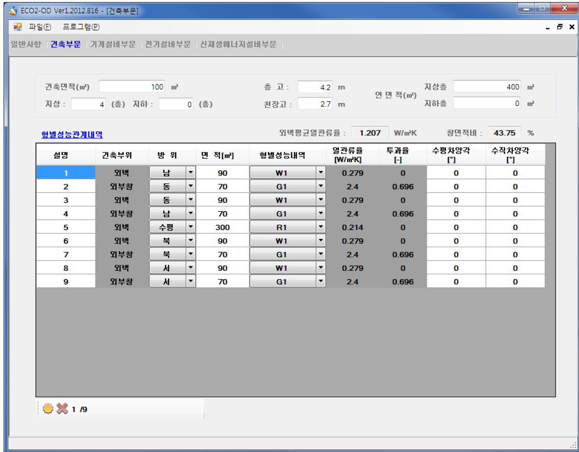
[건축부문 입력화면]
