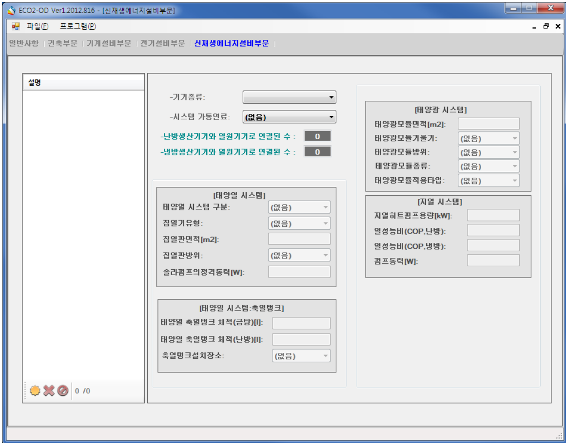
[신재생에너지설비부문 입력화면]
